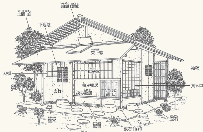
草庵茶室の外観屋根の形
